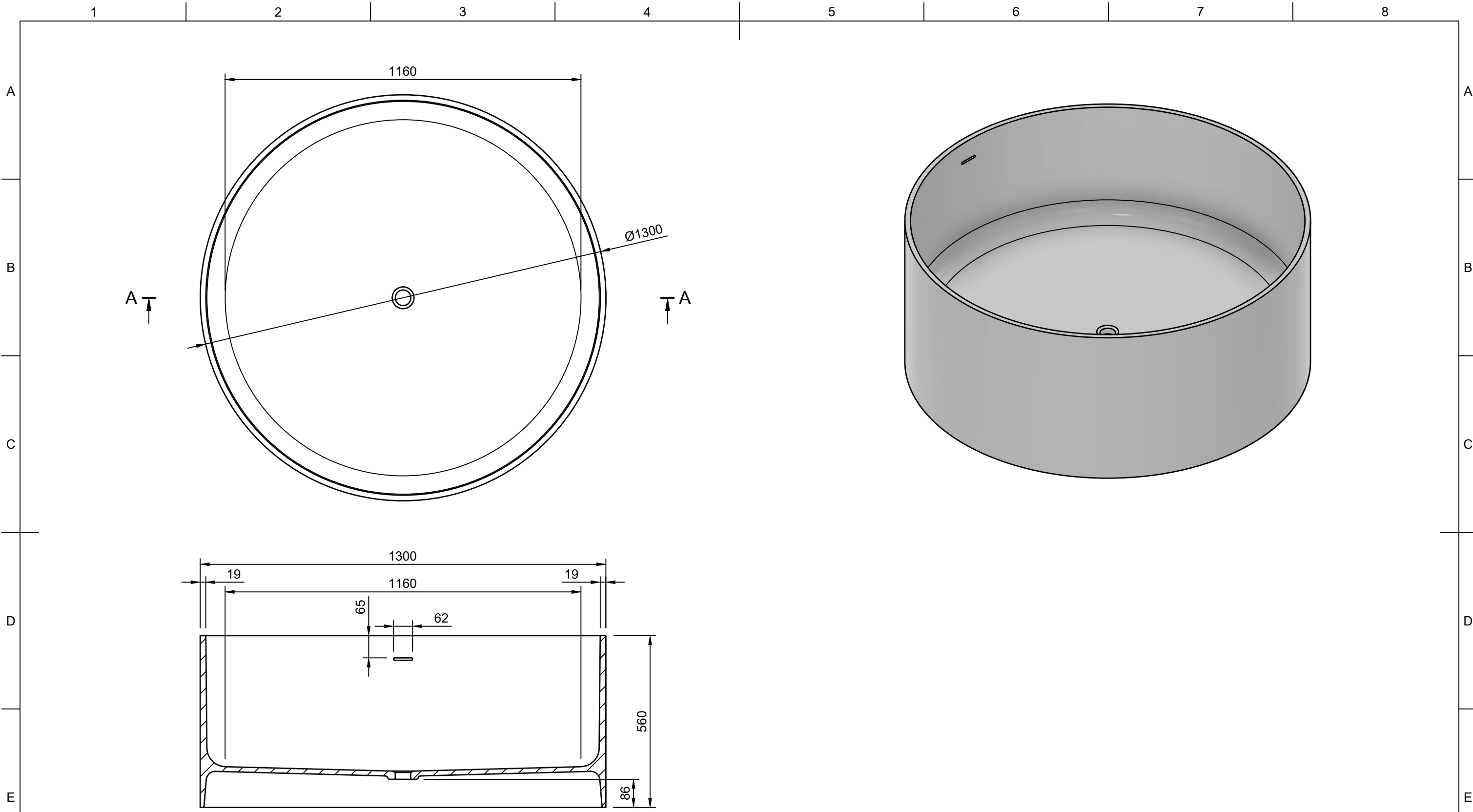
A-A (1:12)
